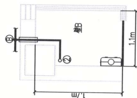
壁挂炉间B入户层天然气管道平面布置图 1:50
